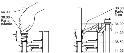
Fig. 4 Montaggio tenuta meccanica
