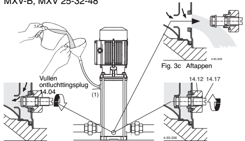
Fig. 3a Vullen: naaldschroef open
