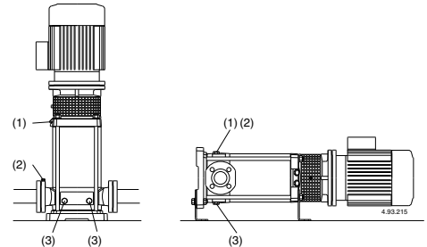
Σχ. 3δ (1) Γέμισμα και εξαέρωση (2) πρόσληψη εξαερισμού (3) Αποστράγγιση
