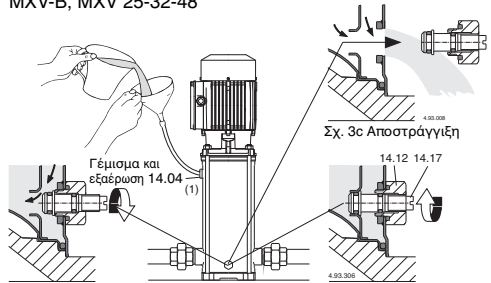
Σχ. 3α Γέμισμα: εσωτερική διόδος ανοίγματος
