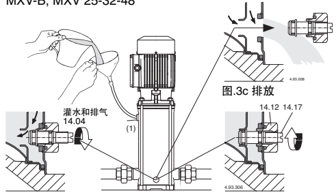
图.3a 灌水: 内部通道打开
