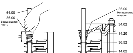
Рис. 5 Установка механического уплотнения
