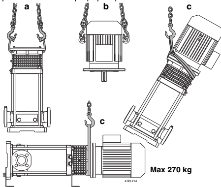
Σχ.1 α Ανύψωση της αντλίας χωρίς μοτέρ β Ανύψωση της κινητήρα χωρίς αντλία γ Ανύψωση της αντλίας με μοτέρ
