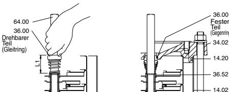
Abb. 5 Montage Gleitringdichtung
