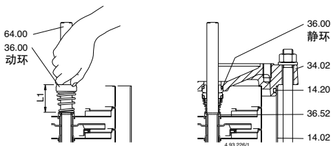
图.4 插入机械密封
