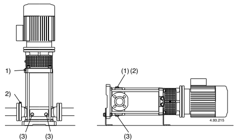
图.3 (1) 灌泵和空气排放 (2) 进口端排气 (3) 排放
