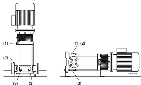
Fig. 3d (1) Riempimento e sfataio (2) Sfataio aspirazione (3) Scarico
