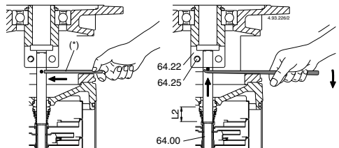
Fig. 5a Rotor posé, arbre non bloqué dans l'accouplement.
