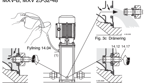
Fig. 3a Fyllning: luftskruv öppen
