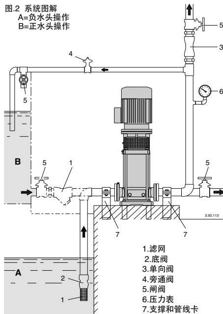
图2 系统图解
