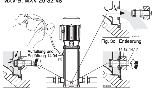
Abb. 3a Auffüllung: Interner Durchgang offen
