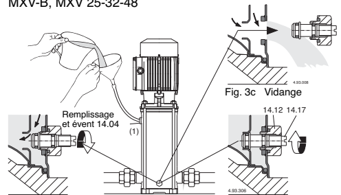
Fig. 3a Remplissage: passage intérieur ouvert
