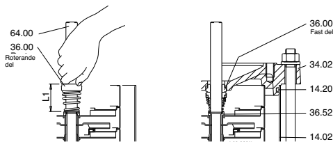
Fig. 4 Montering av axeltätning
