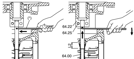
Abb. 5a Stehender Laufer, Welle nicht blockiert in Kupplung (*) Stift für Wellenanheben.
