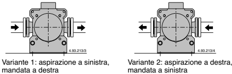
Fig. 6 Orientamento bocche pompa orizzontale
