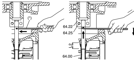
图.5a 转子静止,和轴一起均未被联轴器锁住 (*提升轴用的销
