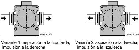
Fig. 6 Orientación de las bocas con la bomba horizontal
