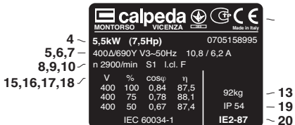
Beispiel Typenschild des Motors, (nur MXV-B)
