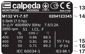
Motorschild - Beispiel 50Hz
